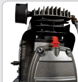
15% más producción de aire Cilindros de hierro fundido. Pistones sobredimensionados para una mayor producción.
